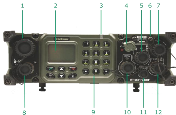
Рисунок 1.10 - Зовнішній вигляд передньої панелі радіостанції VRC 9661.
