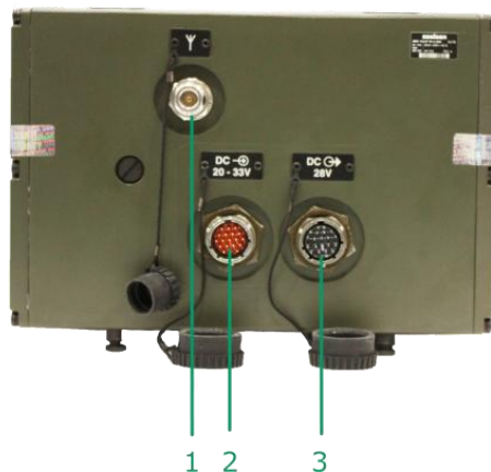
Рисунок 1.15 - Зовнішній вигляд задньої панелі підсилювача потужності на 50 Вт.
