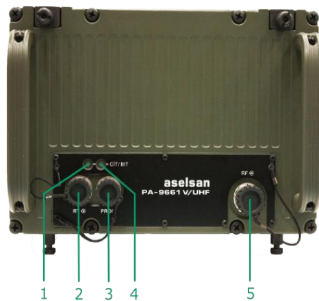
Рисунок 1.14 - Зовнішній вигляд передньої панелі підсилювача потужності 50 Вт радіостанції VRC 9661.
