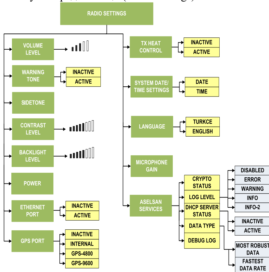
Рисунок 3.26 - Меню налаштувань радіостанції.
